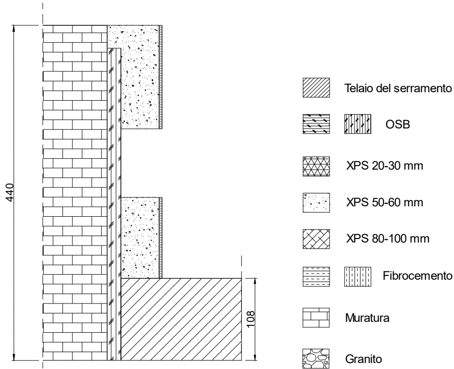
Sezione spalla
