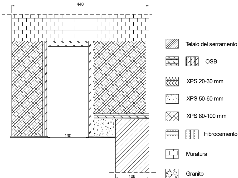
Sezione cassonetto
