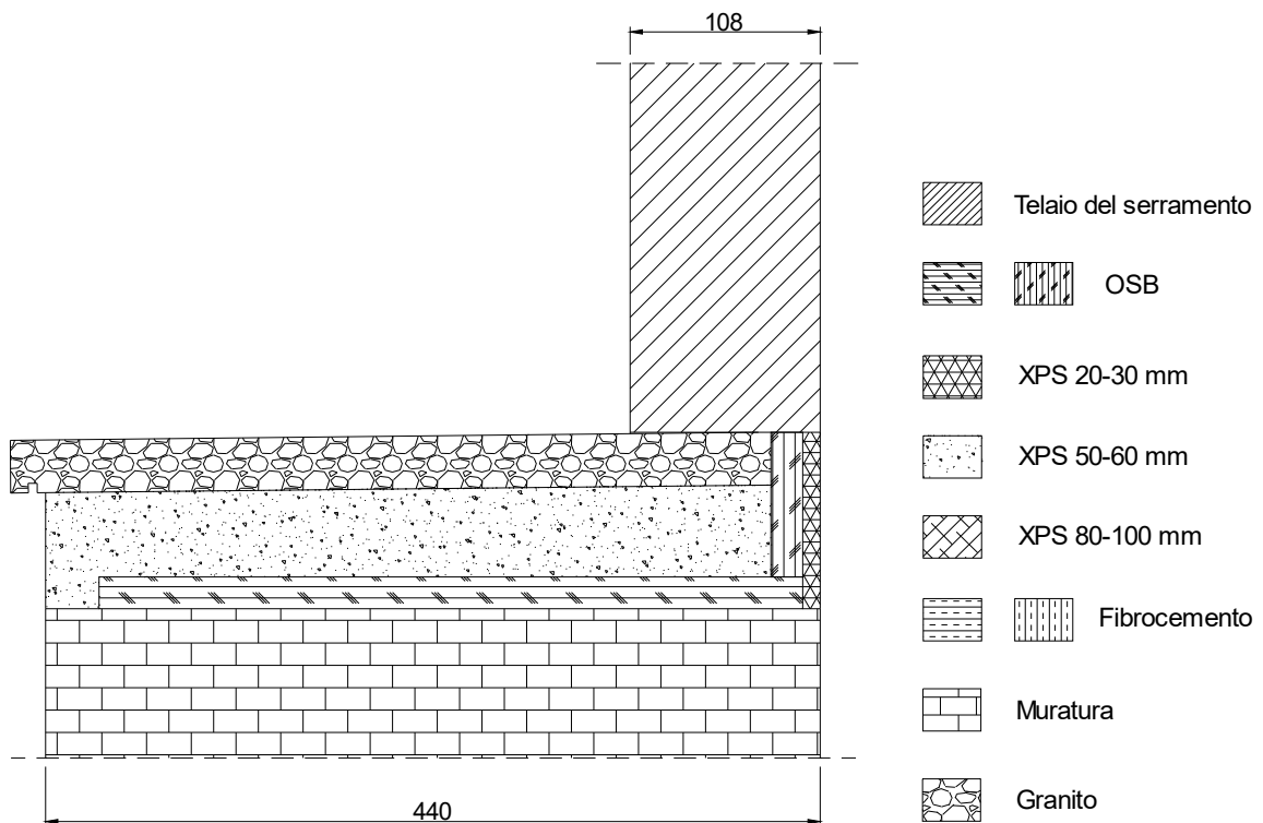
Sezione sottobancale
